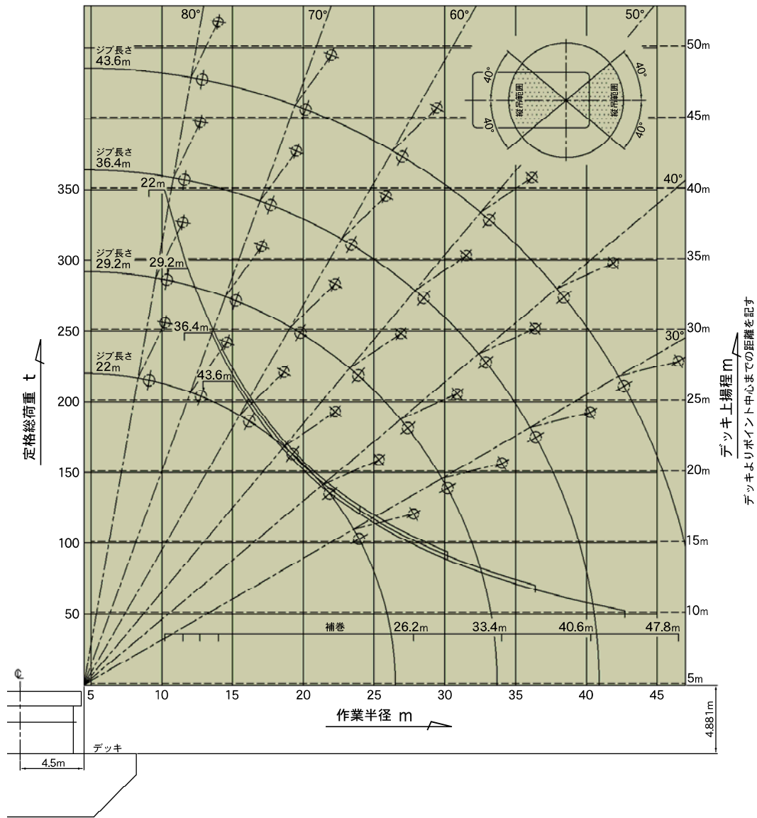
定格総荷重表 350t フック使用時 (総合)
