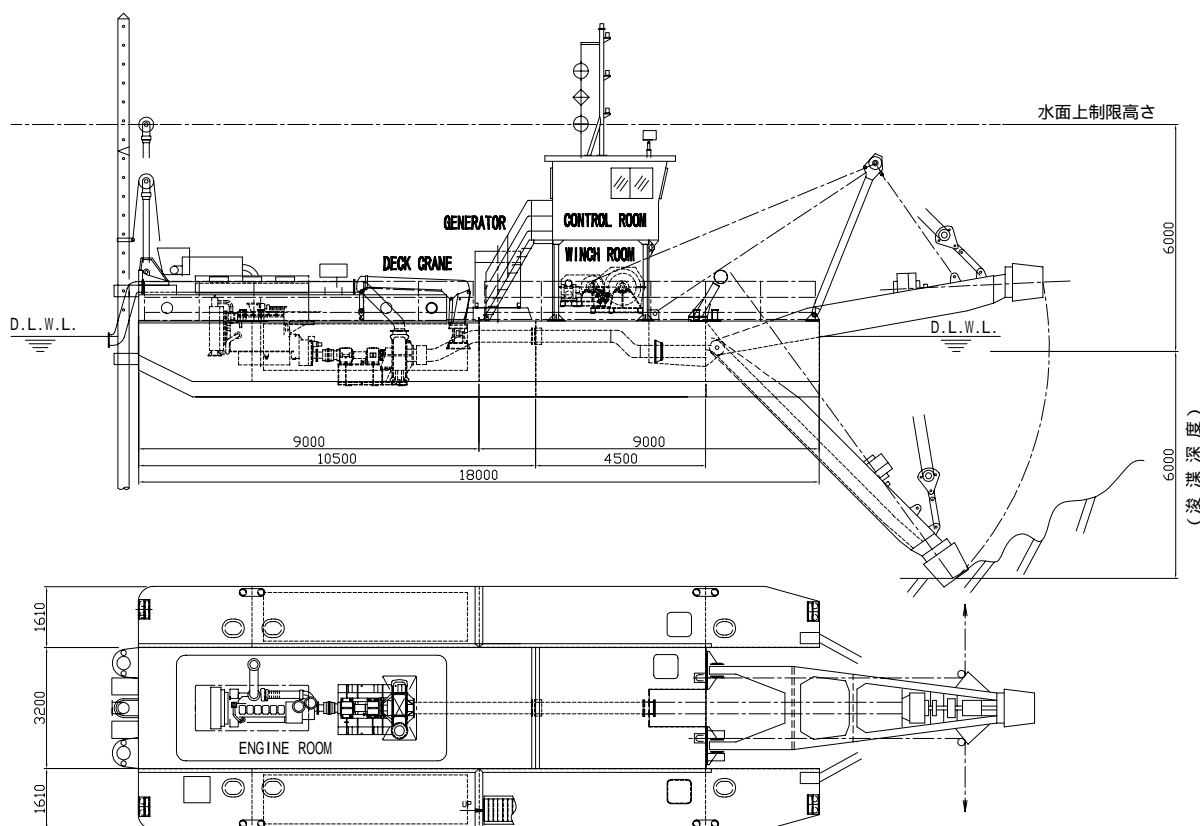
外形図
